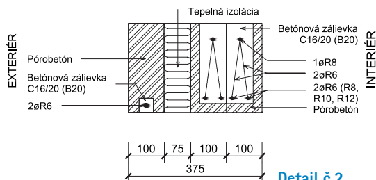
Detail č.2 Zateplený nosný preklad na š. múru 375 mm – kombinácia nosných a nenosného prekladu
